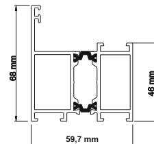
Profil proggu ENERGY 60
