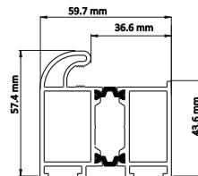
Profil ościeżnicy KMT ENERGY 60
