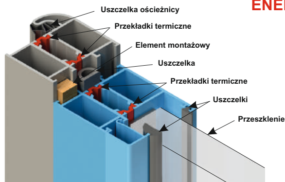
PROFIL OŚCIEŻNICY ENERGY 60
