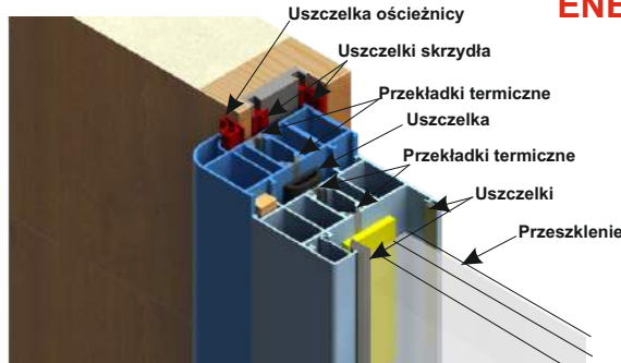
SKRZYDŁO KMT PLUS 75 passive
