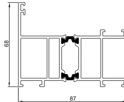
Profil proggu ENERGY 90
